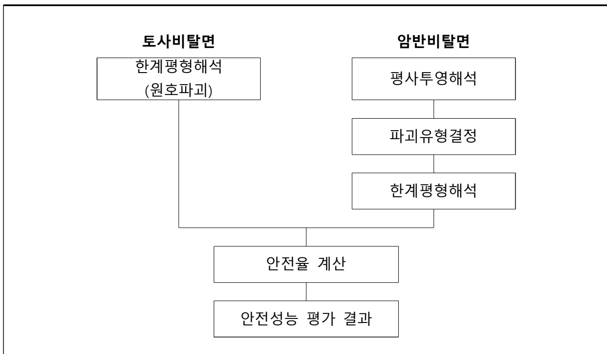
【그림 19.5】 구조안전성능 평가과정
