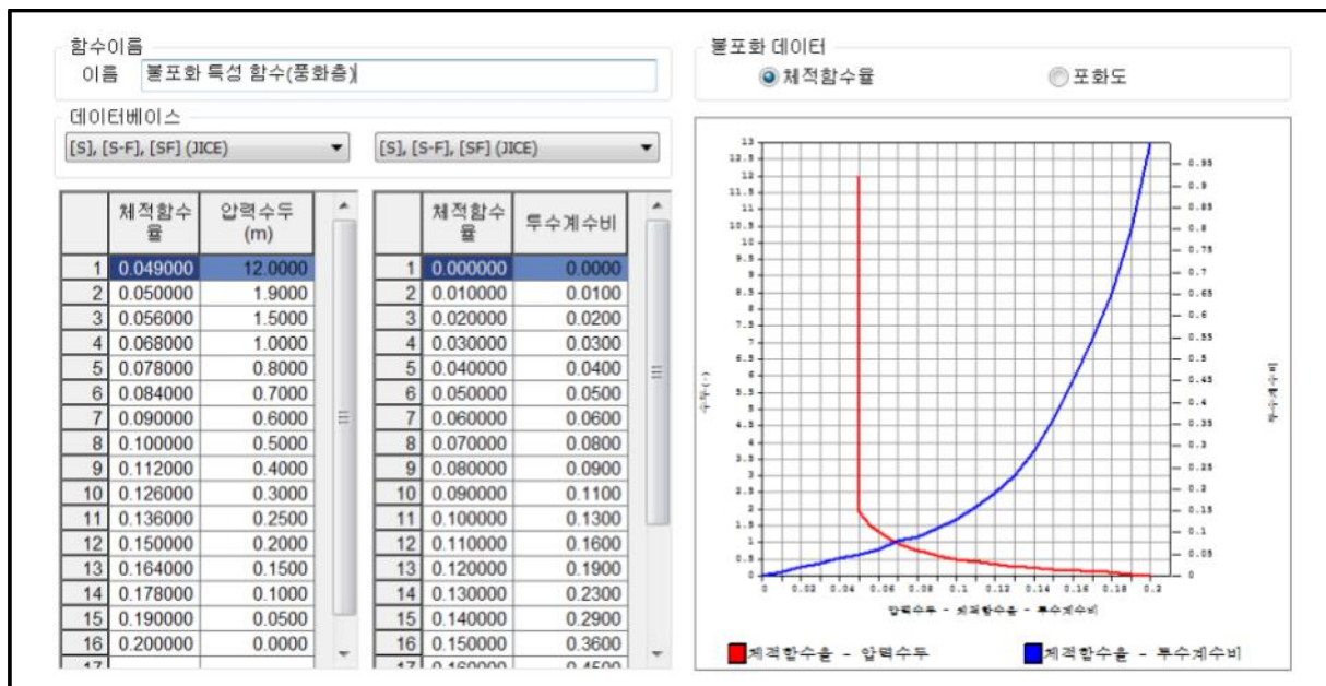
【그림 19.15】 압력수두-채적함수(포화도)-투수계수비 함수
